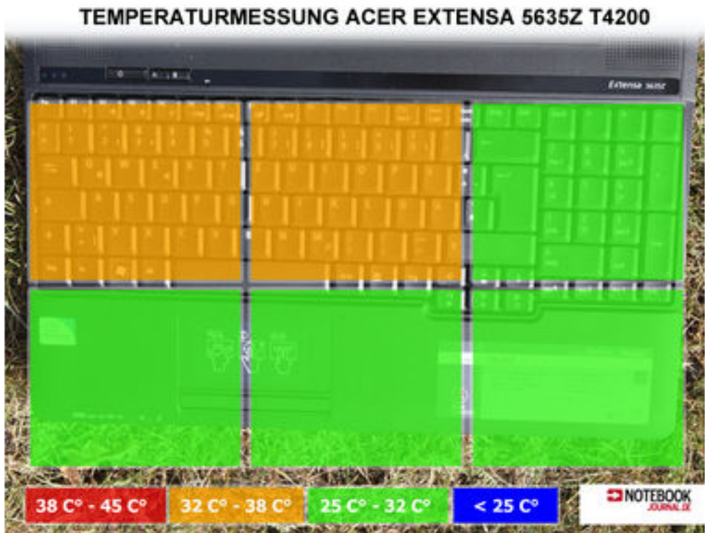
Bild: Notebookjournal/SJ Wärmeentwicklung des Acer Extensa 5635Z-422G16N
